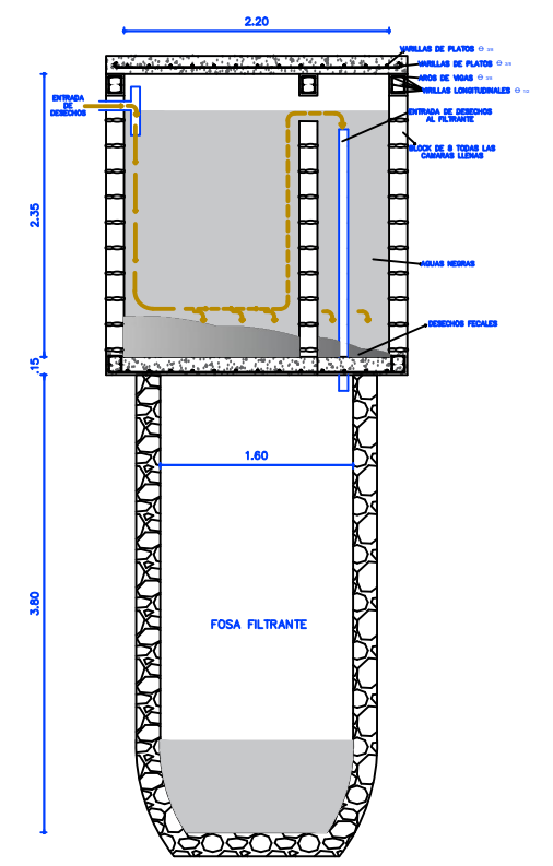
Detalles de sección de septico.
